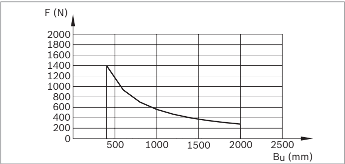
Diagrama 3: carga admisible de la suspensión
