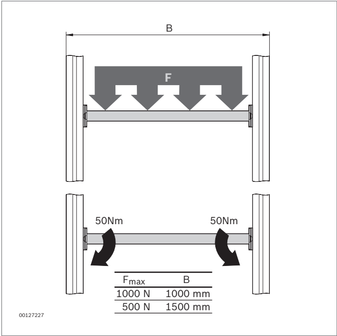
Travesaño tubular con escuadra RTW (página 5-25)
