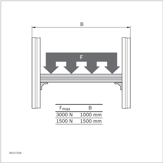
Travesaño de perfil ST (página 5-25)
