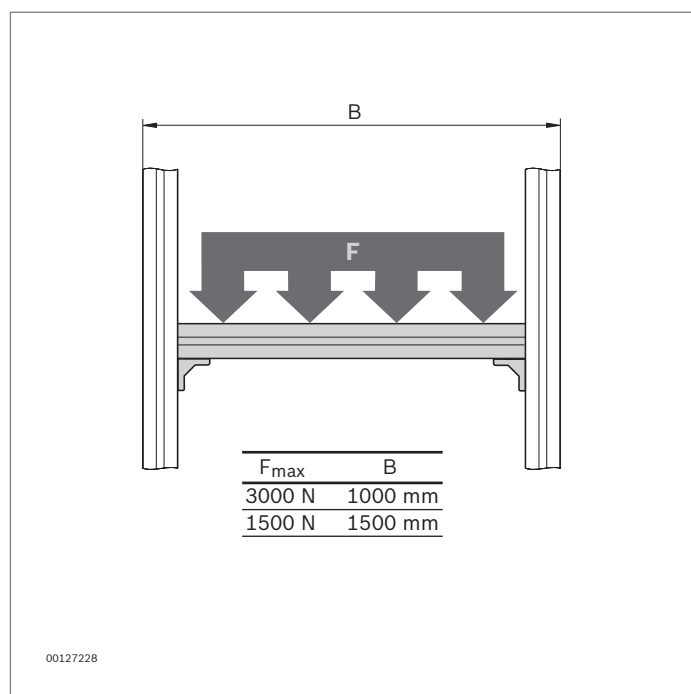
Traversa profilata ST (Pagina 5-25)
