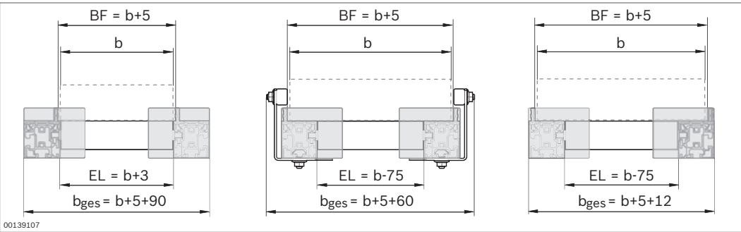
Linea di trasporto EcoFlow con piastra di chiusura
