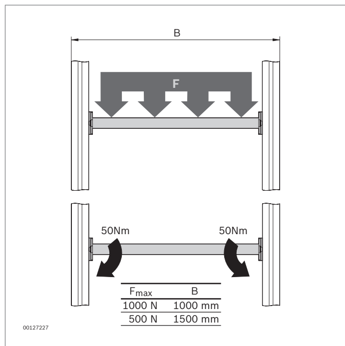
Traverse tubulaire avec équerres RTW (page 5-25)
